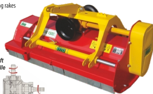
Gearbox extension Halbachse
