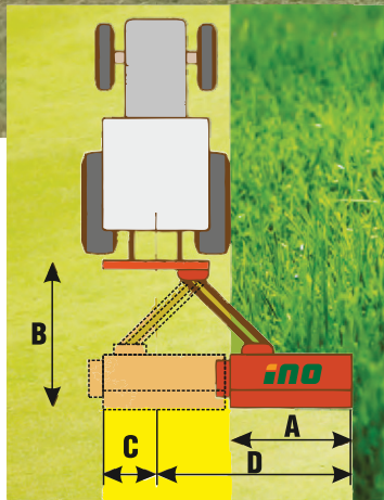
Working position | Arbeitsstellung | Рабочее положение
