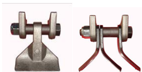
Kladiva standardno, Y noži po naročilu (za lažja opravila).
